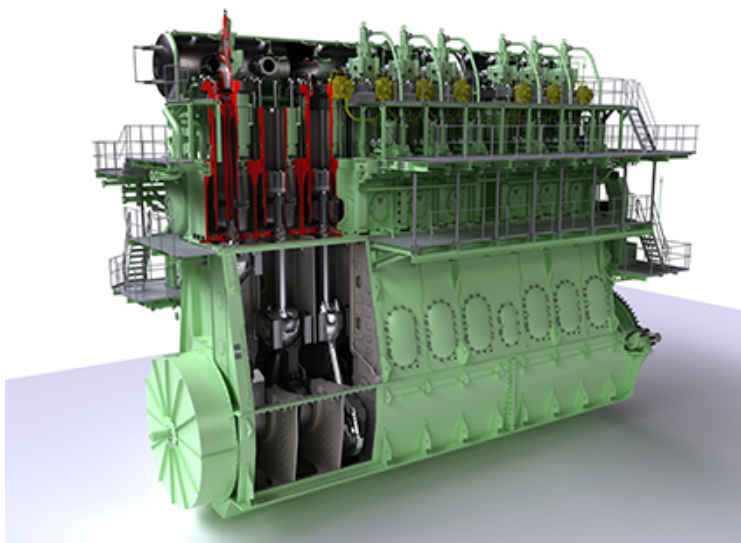
自推出以来，ME-GI 发动机已获订购约 200 台。图中所示为 9S90ME-GI 型发动机
